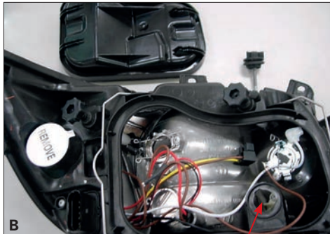
B Die Reflektorhalterung ausbauen.
