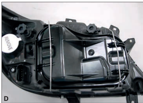
D Abdeckung montieren und Feder einsetzen.
