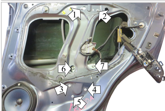
POWER WINDOW RIGHT ALZACRISTALLI ELETTICO DX
