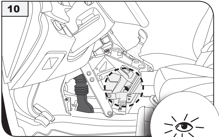
Gehäuse 16pin OBD connector 16pin OBD
